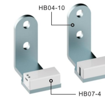
Assembly diagram 组装图
